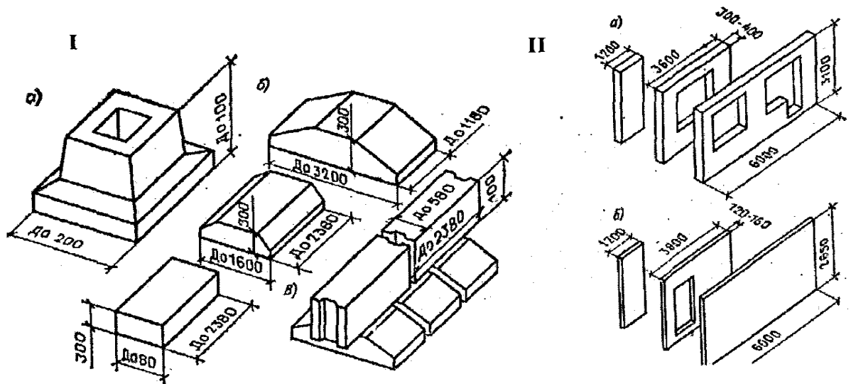
Сурет 1. Азаматтық үйлер құрылысында қолданатын кейбір темірбетонбұйымдары: I – іргетас элементтері: а – сатылық іргетас блогі; б – жертөле қабырға блогі; в – бағана астына іргетас; II – тұрғын үй панельдері: а-сыртқы қабырға панельдері; б- ішкі қабырға панельдері
